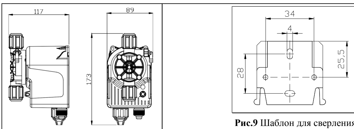
Рис.8 Габаритные размеры
